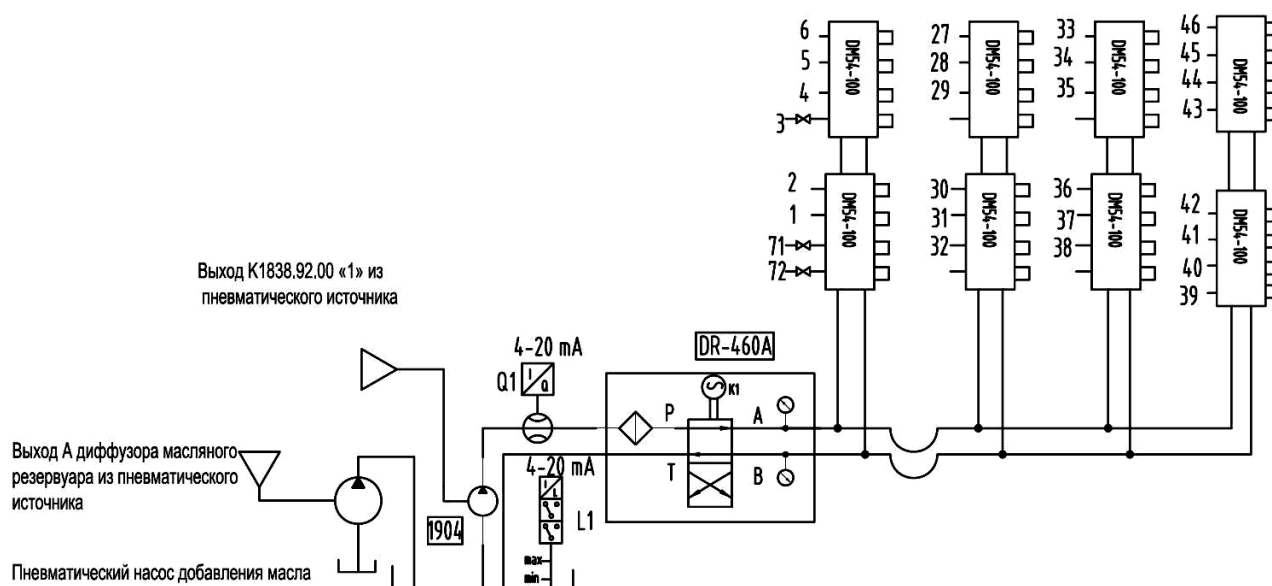
Рисунок 1. Схема смазки верхней части экскаватора WK-35
