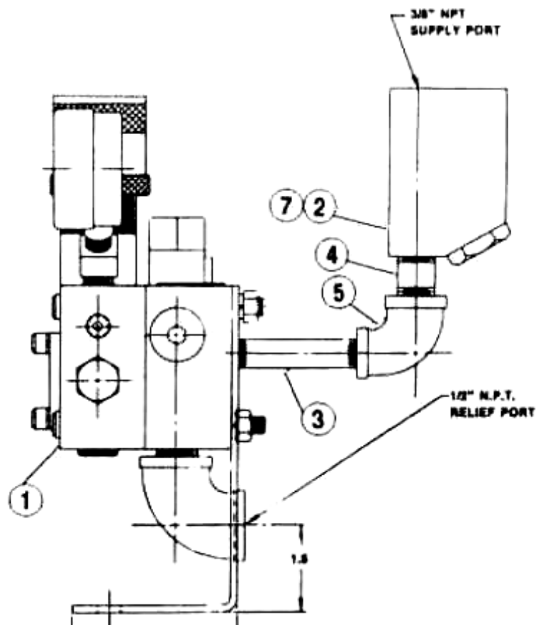
Рисунок 15. Схема гидрораспределителя DR-460В
