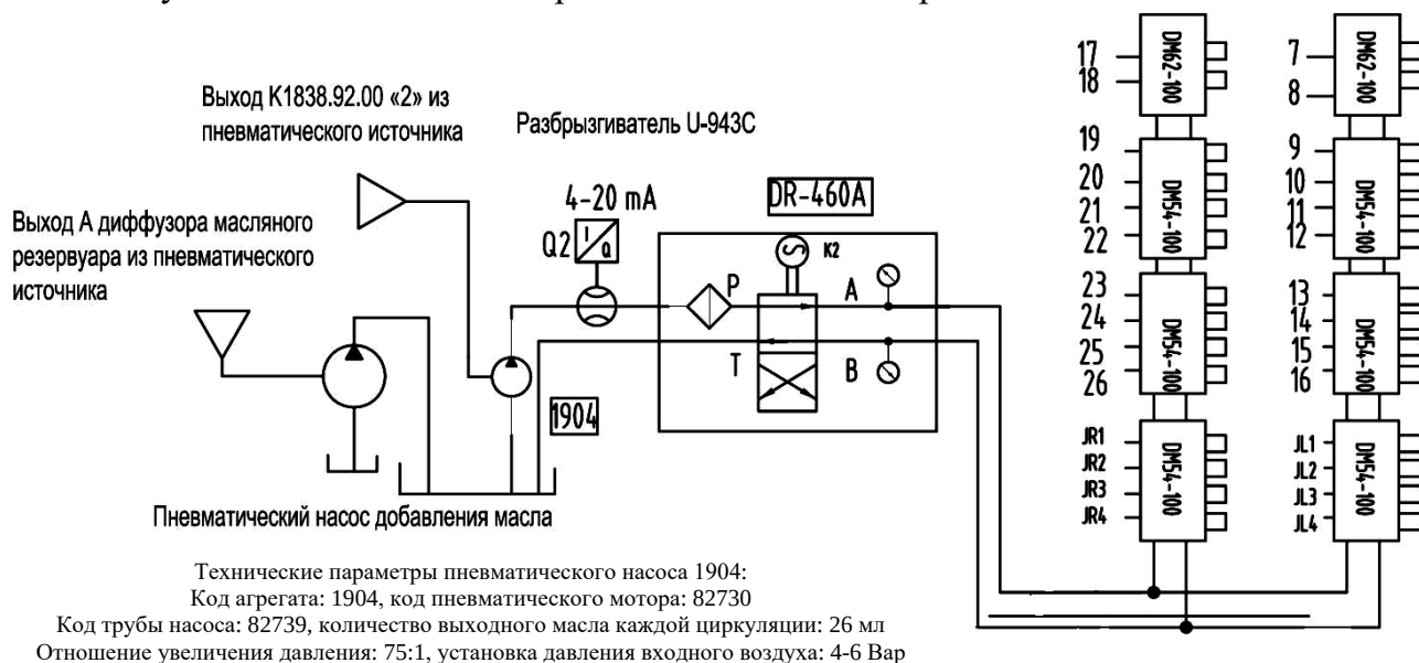
Рисунок 2. Схема смазки нижней части экскаватора WK-35
