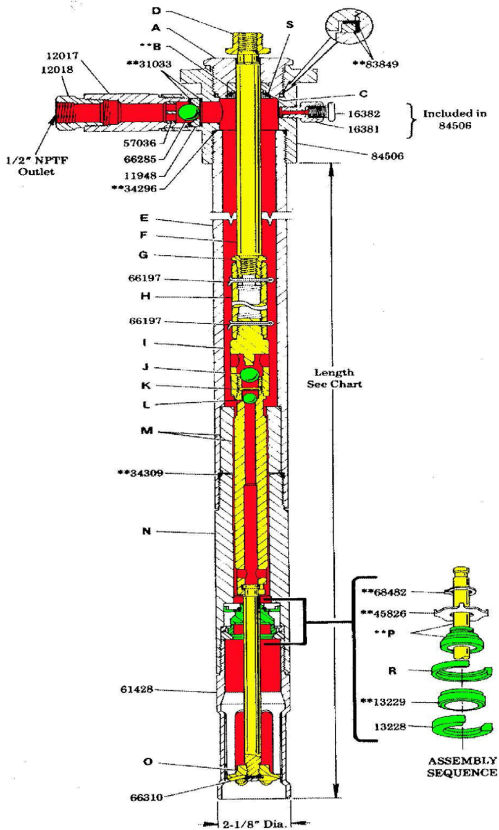
Рисунок 12. Схема насосной трубы 82793
