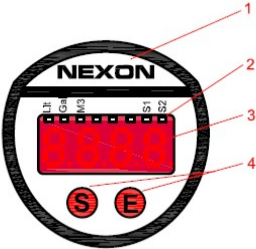
Рисунок 22. Дисплей расходомера
