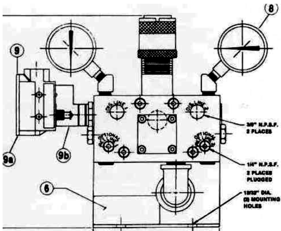
Рисунок 15. Схема гидрораспределителя DR-460В
